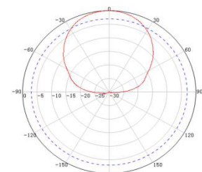
V-Plane
