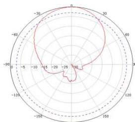
H-Plane
