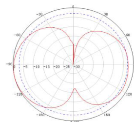
V-Plane
