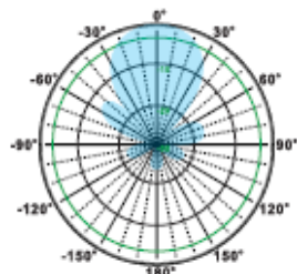
V-Plane
