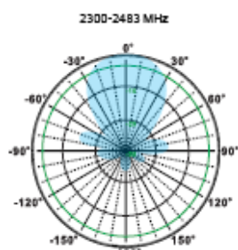
H-Plane
